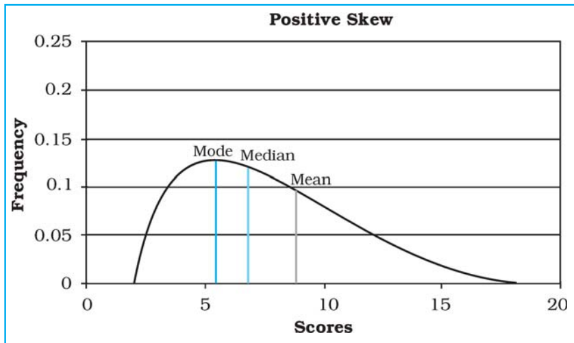
Fig. 2.4 : Positive Skew
